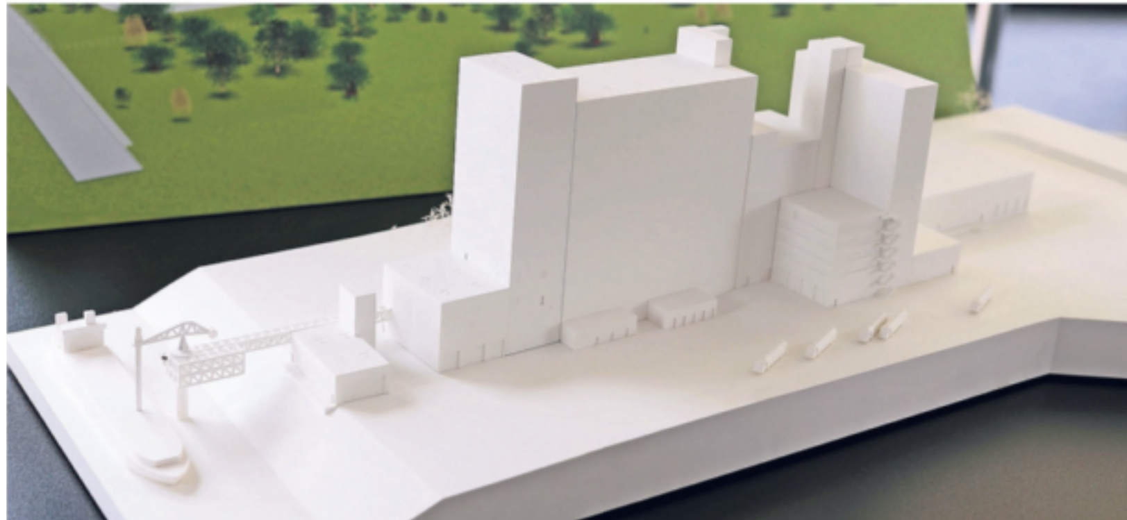
In dem Modell ist die Anlegestelle für Binnenschiffe und das Gleis für den Transport von Roggen und Weizen mit der Hafenbahn zu erkennen. RP-FOTOS (2): LAMMERTZ
